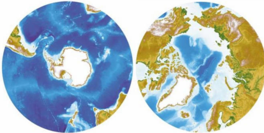
Abbildung: Topografische Karten für Antarktis (links) und Arktis (rechts)
